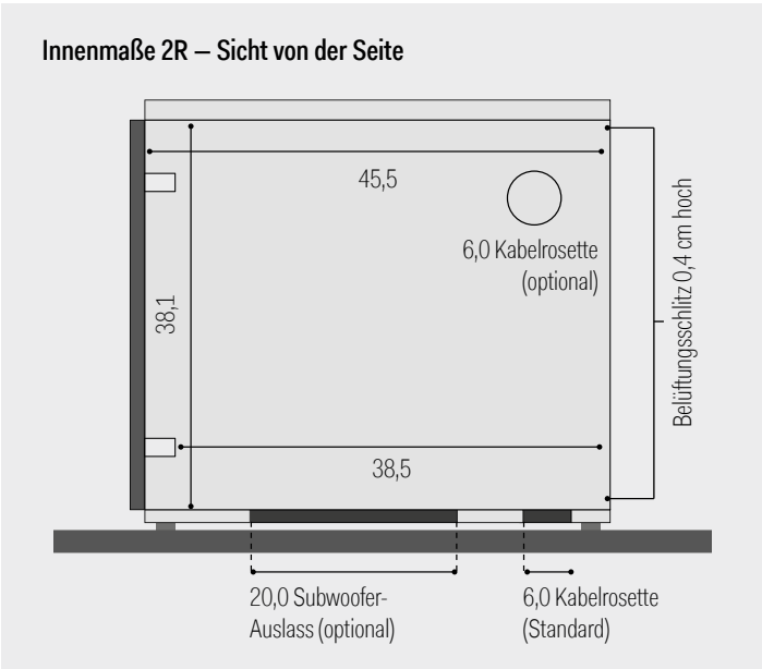
Akustikstoff und Rückwand, Schwarz, Innenseiten und -böden in Korpusfarbe.
